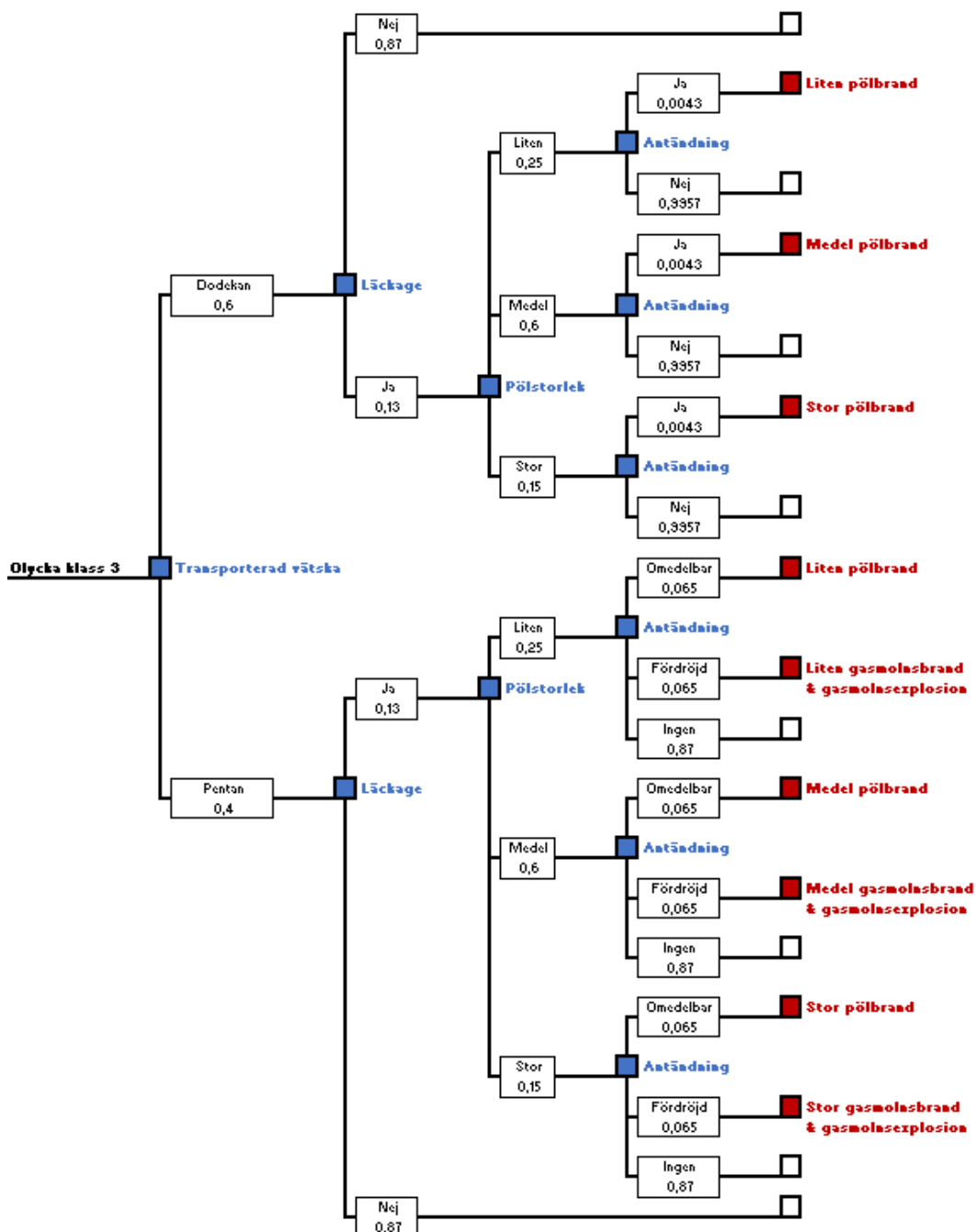
Figur 5-5. Händelse-träd för olycka med brandfarlig vätska.
