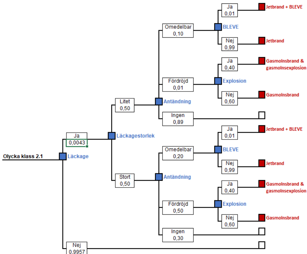
Figur 5-2. Händelsetråd för olycka med brandfarlig gas.
