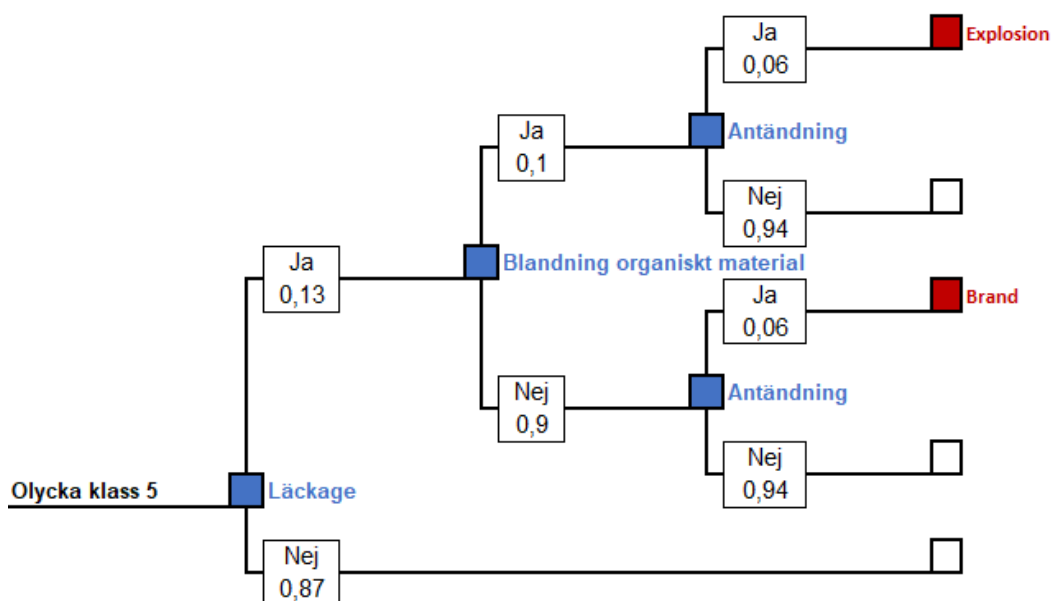
Figur 5-6. Händelseträäd för olycka med oxiderande ämnen och organiska peroxider.
