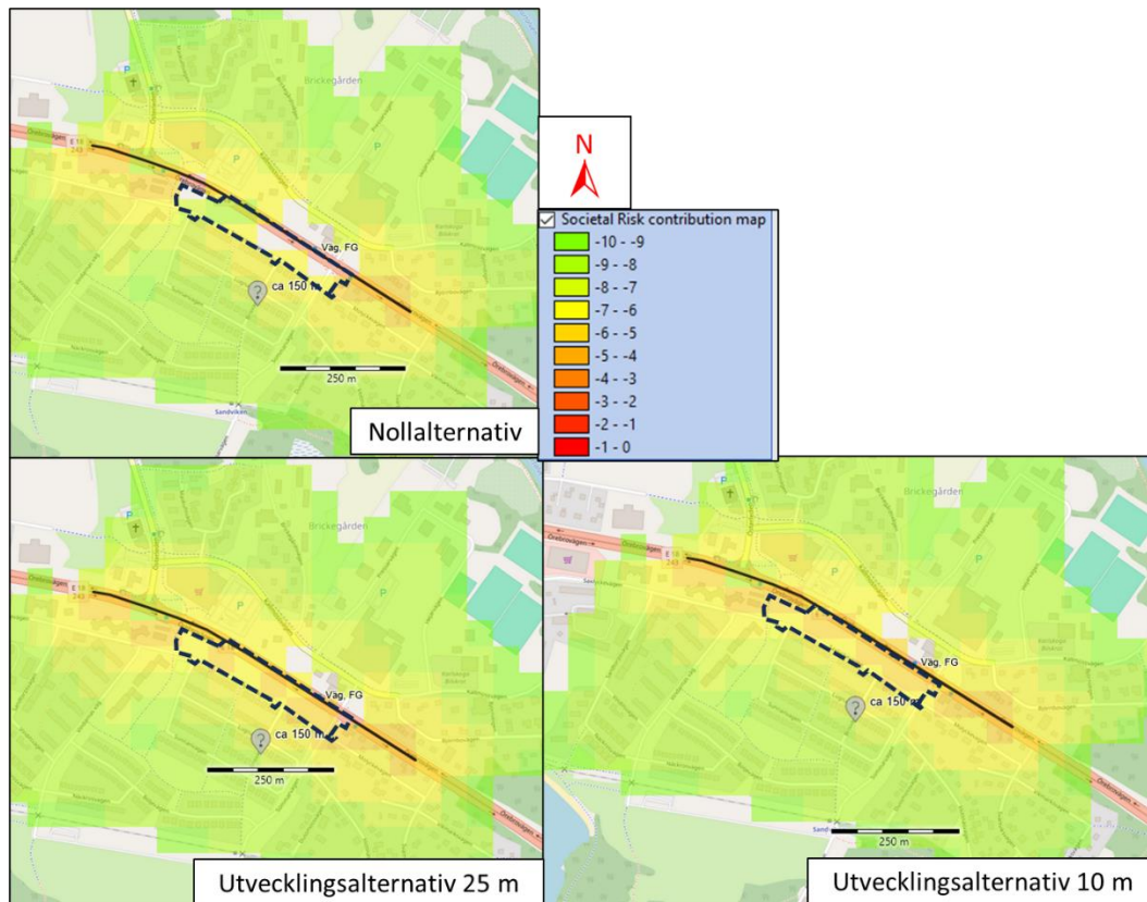
Figur 6-6. Planområdet och närmsta omgivningarnas bidrag till samhällsriskenivån. Färgerna symboliserar det relativa bidraget och går i skala från röd-orange-gul-grön (högst till lägst bidrag) där ingen färg betyder inget bidrag till samhällsrisken.
