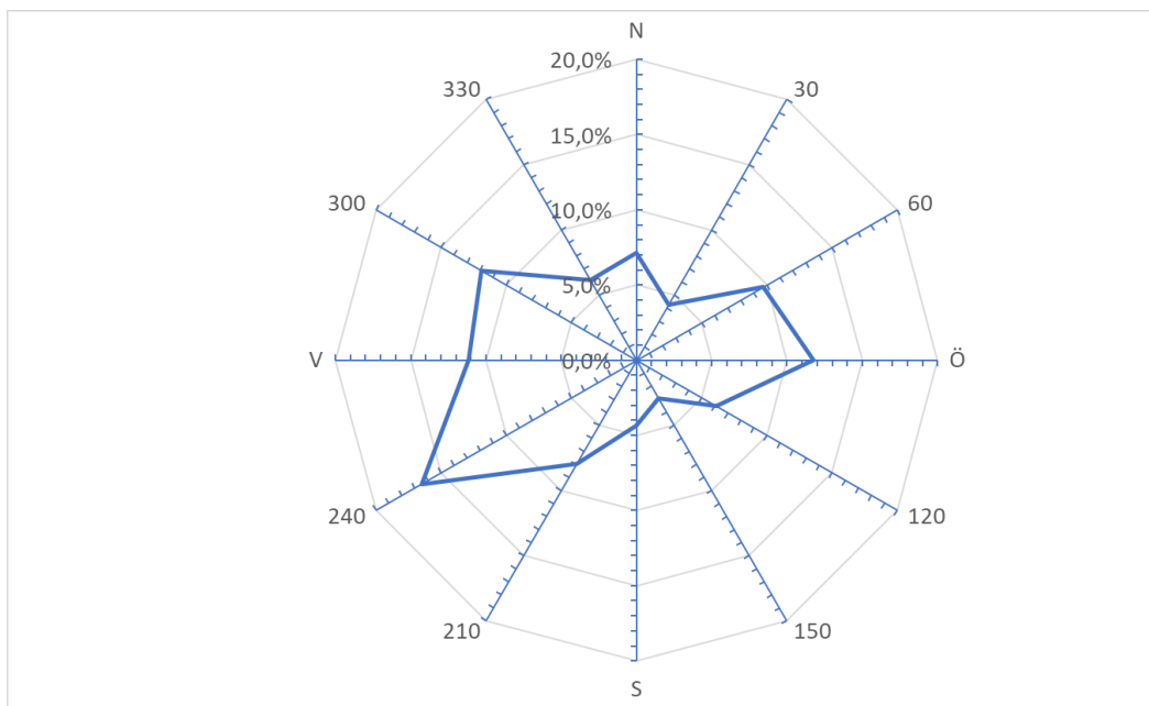
Figur 4-3. Fördelning av vindriktning vid mätstation Kilsbergen-Suttarboda A, år 2004 – 2024.
