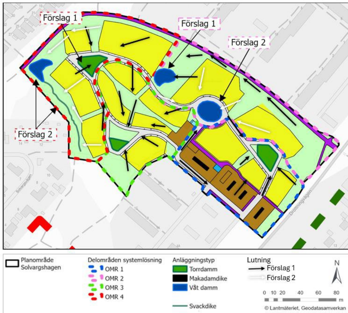
Figur 31: Föreslagen systemlösning inom planområdet Solvargshagen. Dammarna är skalenliga, diket och makadamdikena är ej skalenliga.
