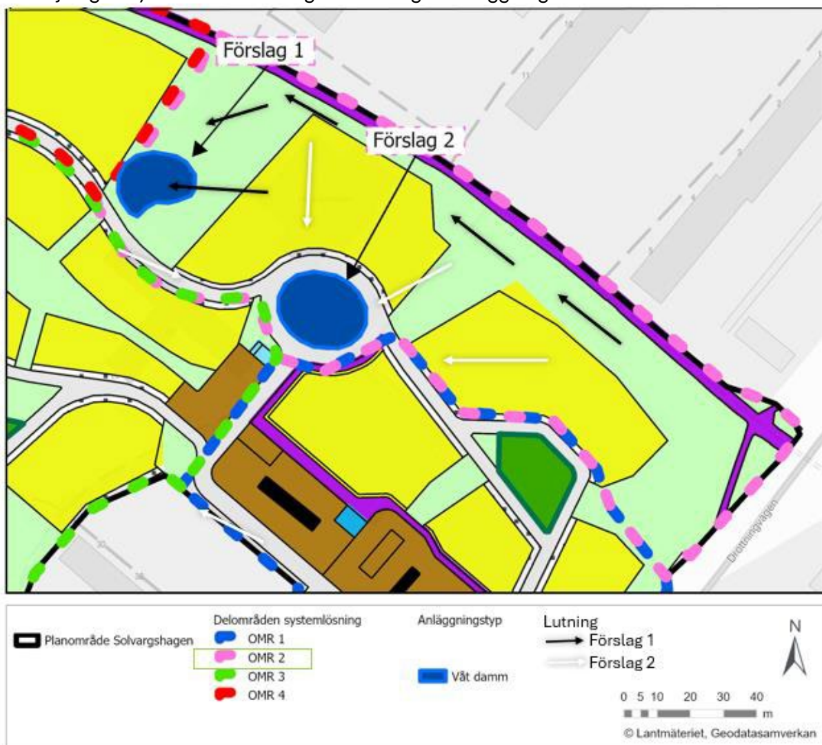
Figur 33: Inzoomad bild över föreslagna systemlösning inom OMR 2 (lila). Anläggningarna är skalenliga.
