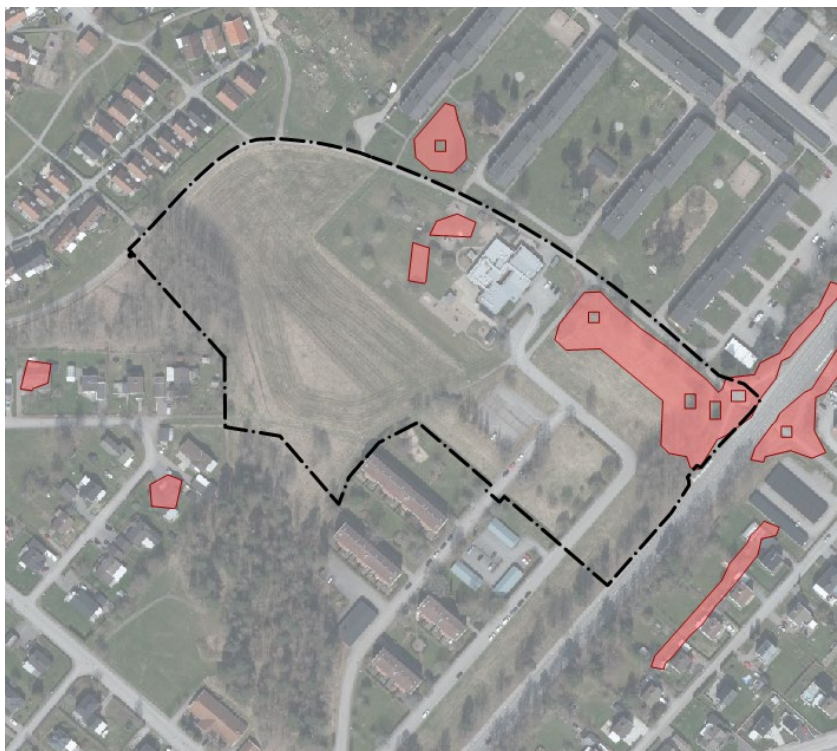
Figur 18: Ras- och skredriskområden – röda ytor. Planområdet – svart-streckad linje.
